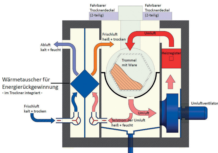
Trocknungsprozess im Galvadry® mit integrierter Energierückgewinnung
